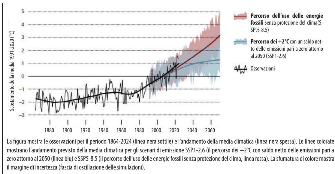
Immagine 1. Evoluzione della temperatura media annuale in Svizzera (Fonte: Clima CH2025, MeteoSvizzera, p. 17)
